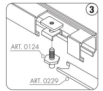
Вставить верхний болт ART. 0124 и закрутить его при помощи регулировочного ключа ART. 0229.
