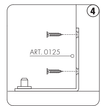
Прикрутить монтажную скобу ART. 0125 к дверной коробке.
