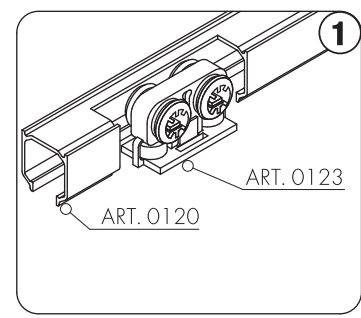
Вставить верхний ролик ART. 0123 в алюминиевый профиль ART. 1020.
