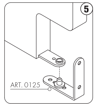
Установить дверное полотно на нижний уголок ART. 0125.
