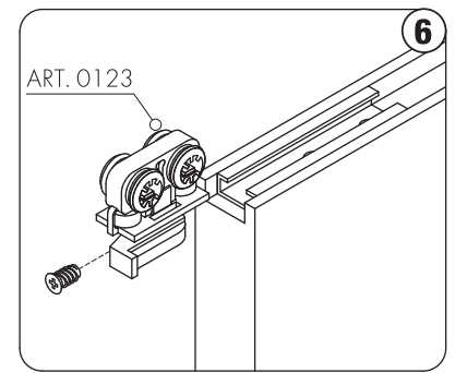
Установить верхний ролик ART. 0123 в сборе с бегунком в алюминиевый держатель и закрепить при помощи «евровинта».
